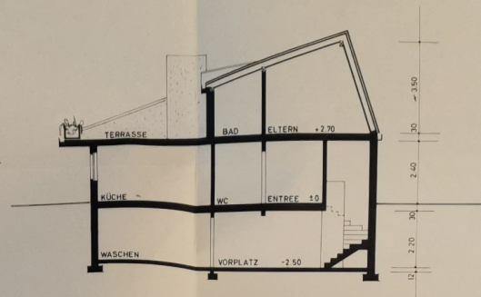
SNITT A-A
