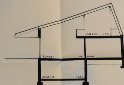
SNITT B-B
