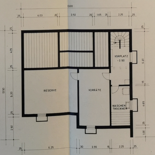
KELLERGESCHOSS
