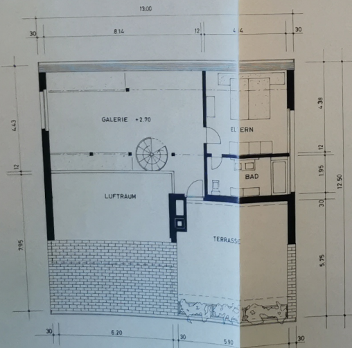
DACHGESCHOSS
